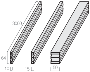
FS610 FS615 FS650 GETO-64 Heavy-Duty Supplementary Panel 志特 -64 重型补充模板
