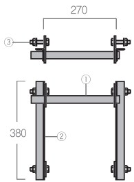
CH-2A Hook 吊钩 ① Main Component ① 主部件 ② Accessories ② 辅件 ③ Hexagon bolt and nut ③ 六角螺栓和螺母
