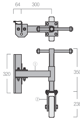
CP6-SC200A Column formwork roller component Used For GETO-64 Heavy-Duty Type 柱模板滚轮组件 用于志特 -64 重型
