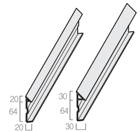
CS620 CS630 GETO-64 Heavy-Duty Corner Correction 志特 -64 重型角部修正条
